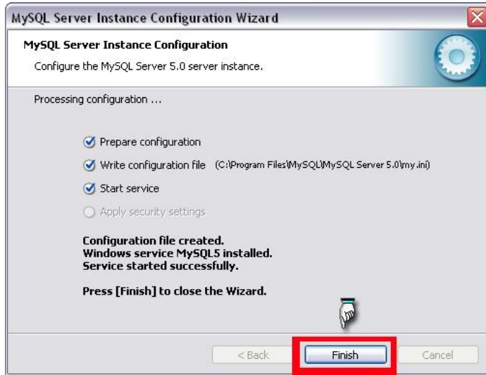
Şekil 2.13 Yapılandırılmanın bitirilmesi
