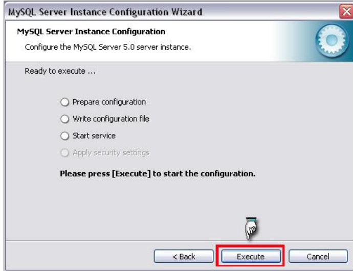
Şekil 2.12 Yapılandırılmanın çalıştırılması
