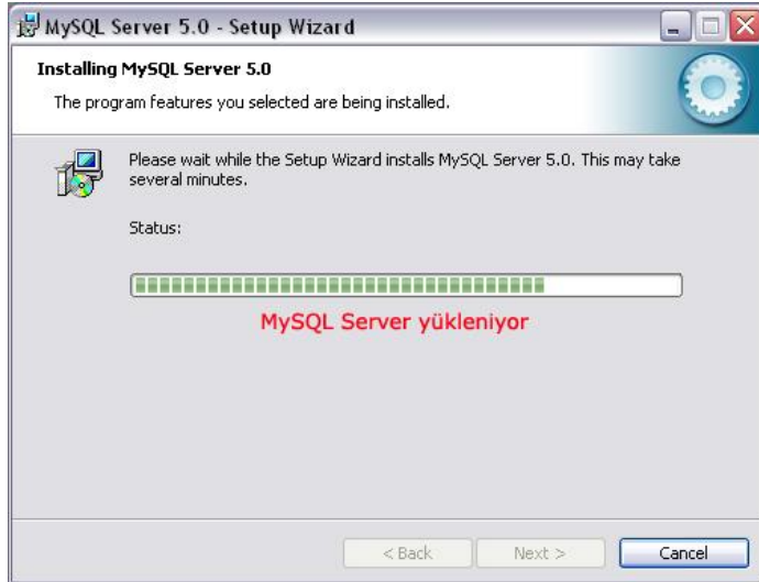
Şekil 2.5 Veritabanının yüklenmesi
