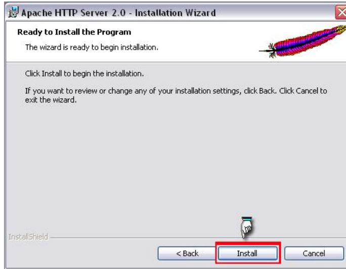
Şekil 1.9 Kurulum başlanması
