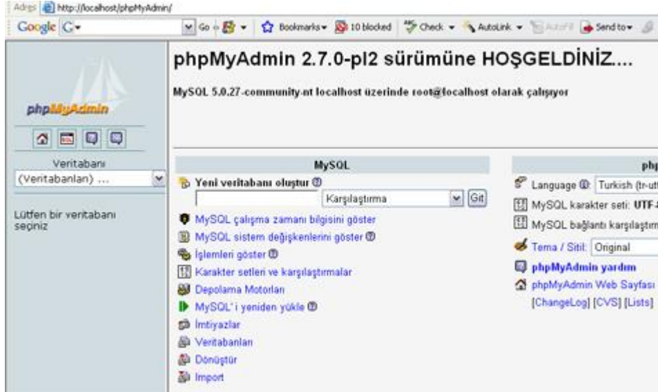
Şekil 2.19 phpmyadmin penceresi
