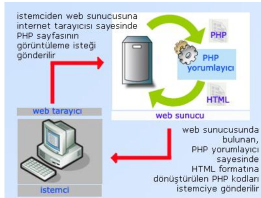
Şekil 1.1 PHP çalışması
