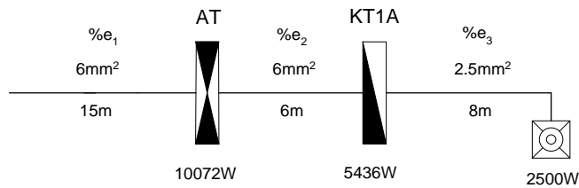
Şekil 3.8: Gerilim düşümü ve akım kontrolü için kullanılacak örnek tek hat şeması
