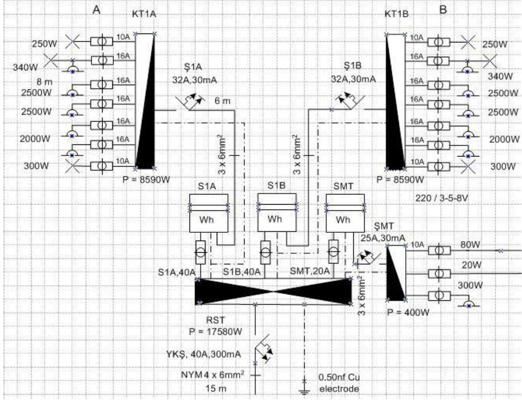
Şekil 2.10: Bir örnek kolon şeması
