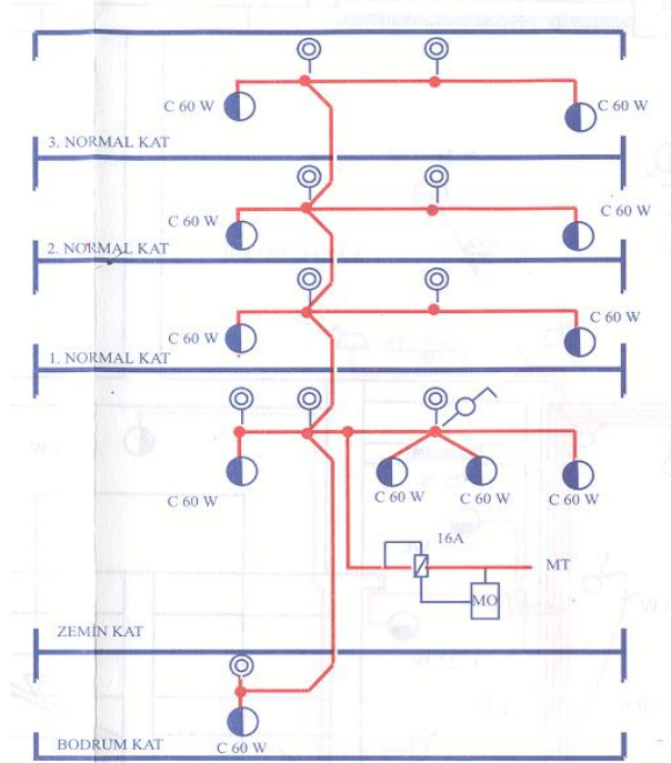
Şekil 3.3: Örnek bir merdiven otomatığı kolon şeması
