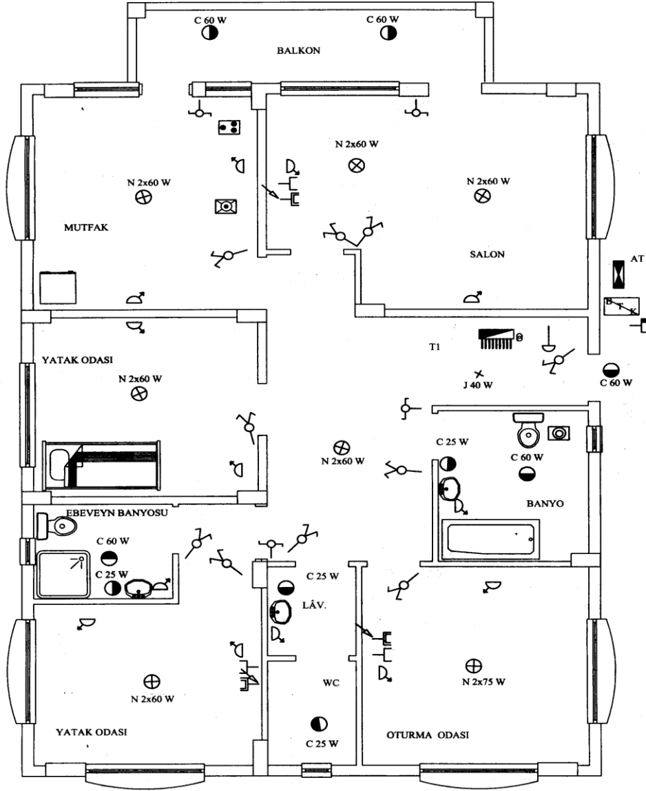
Şekil 2.8: Örnek bir evin anahtar ve prizlerinin yerleşimi
