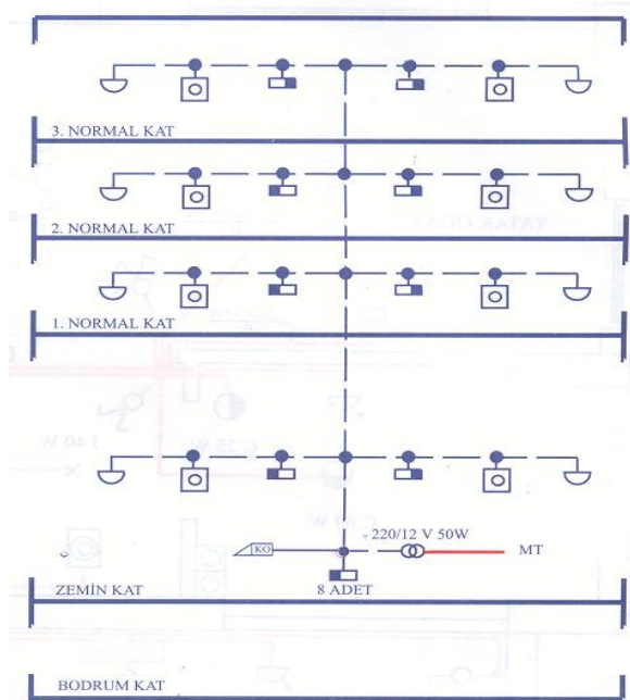
Şekil 3.6: Örnek bir zayıf akım kolon şeması
