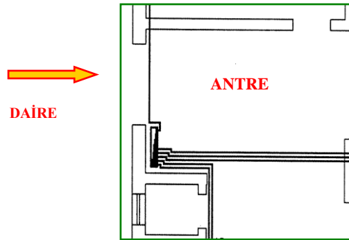
Şekil 2.7: Dağıtım tablosunun yerleşimi
