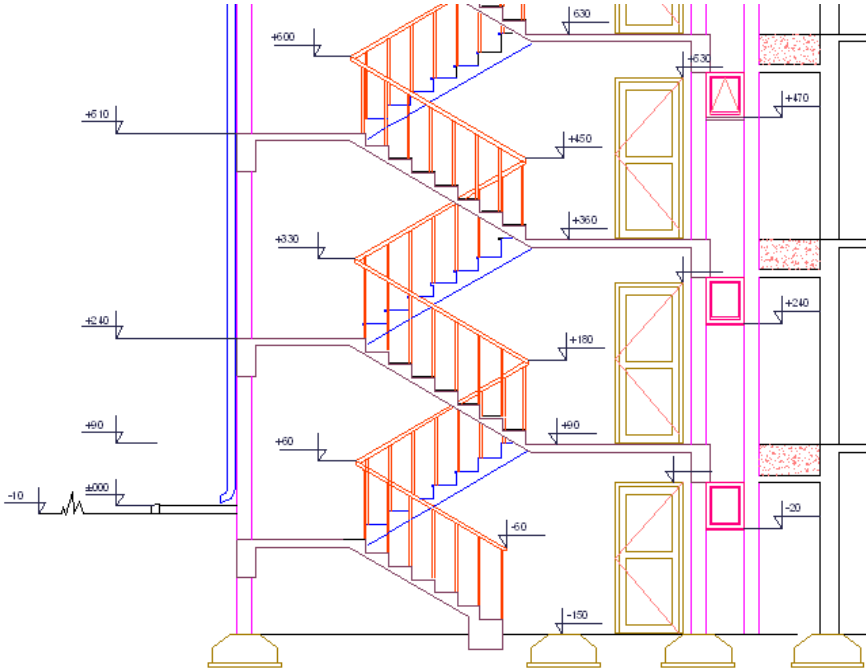
Şekil 1.16: Kesitte kotlu ölçülendirme
