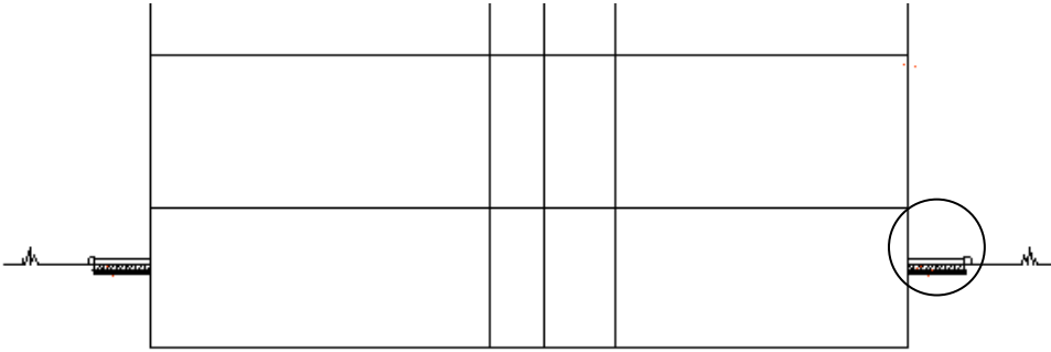
Şekil 1.2: Zemin ve tretuvar çizimi
