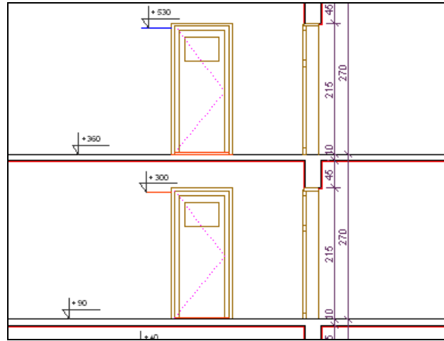
Şekil 2.13: Kotlu ölçülendirme
