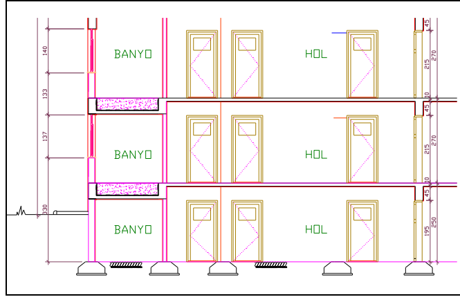
Şekil 2.12: Kesit ölçülendirme
