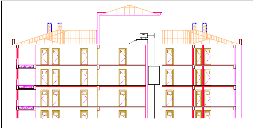
Şekil 2.9: Çatı çizimi
