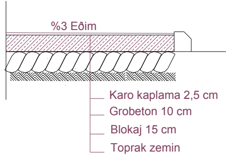
Şekil 1.2: Zemin ve tretuvar çizimi
