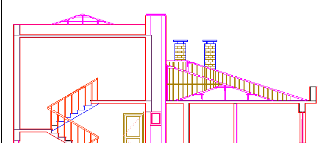
Şekil 1.13: Baca çizimleri
