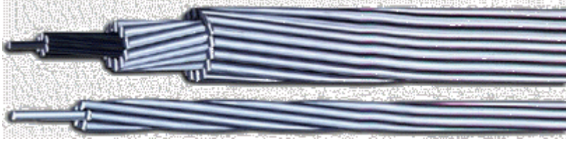
Resim 1.29: Çelik özlü alüminyum iletken (St-Al)
