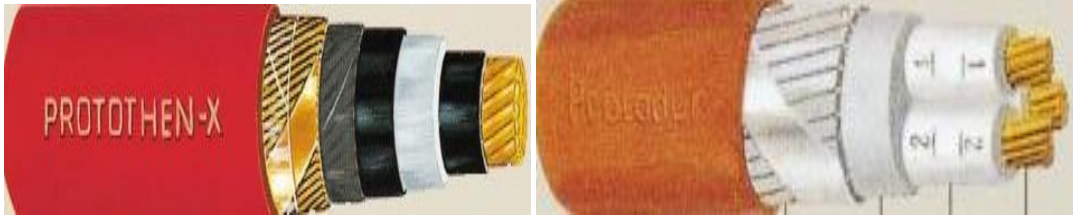
Şekil 2.1: Protothen-x ve protodur yalıtkanlı kablo
