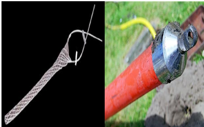
Resim 2.7: Kablo çekme için çorap ve kablo ucu
