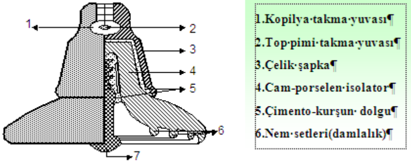
Şekil 1.10: Zincir tipi izolatör yapısı
