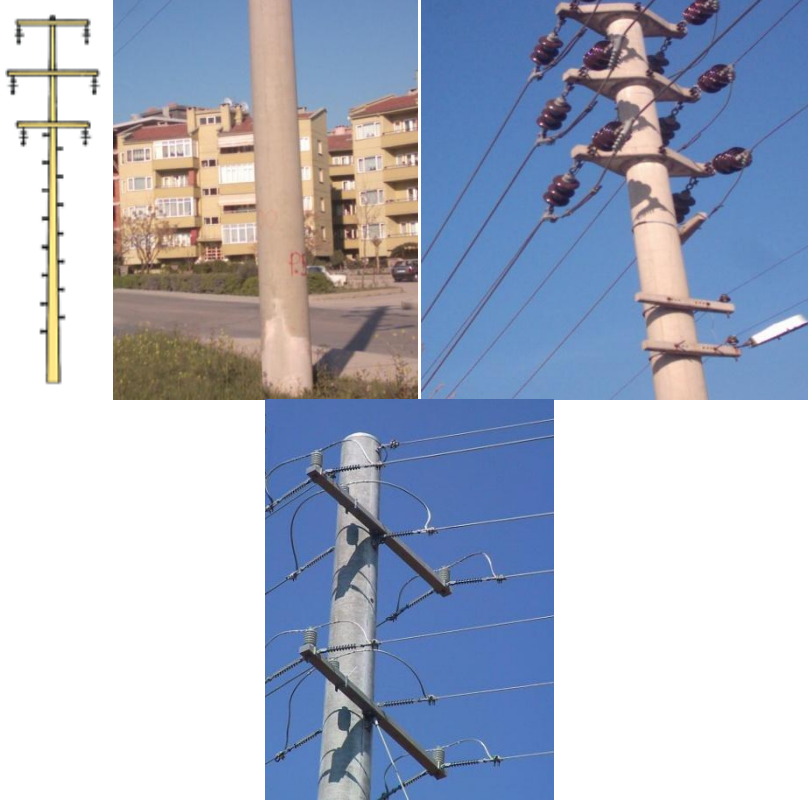
Resim 1.8: Santrifüj (SBA) yuvarlak tip beton direkler
