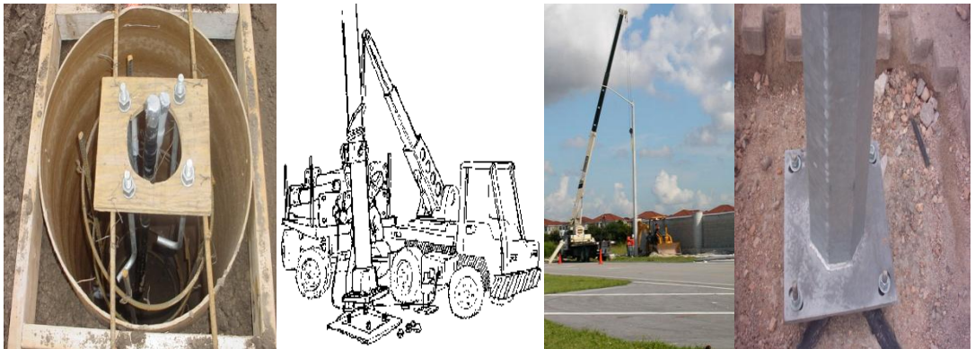
Resim 1.6: Boru tipi direğin yerine montajı
