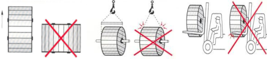
Şekil 2.8: Kablo makarasının taşınma yöntemleri
