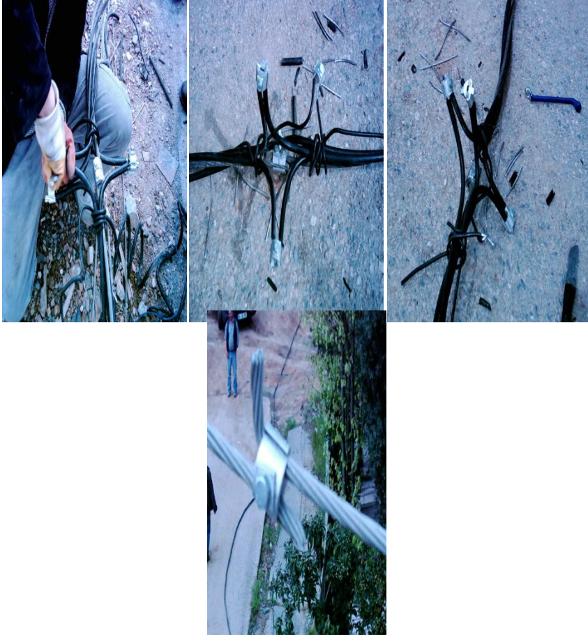
Resim 1.35: Alpek iletkenlerin klemensle eklenmesi
