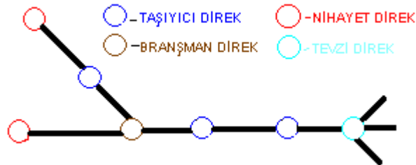
Şekil 1.7: Direklerin yerleşimi
