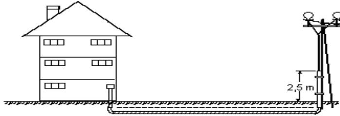
Şekil 2.13: Yer altından enerji girişi
