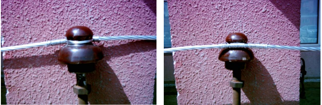
Resim 1.36: İzolatöre iletken bağlantı yöntemi
