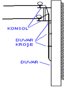
Şekil 1.14: Duvardan açık konsol ile enerji girişi
