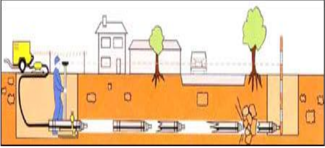
Şekil 2.11: Yer altından kanal açma yöntemi
