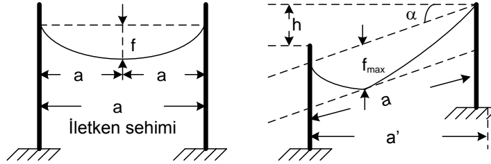
Şekil 1.12: Sehim (fleş)
