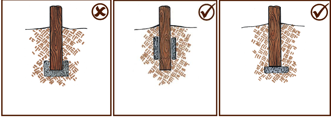
Şekil 1.2: Ağaç direk temelleri
