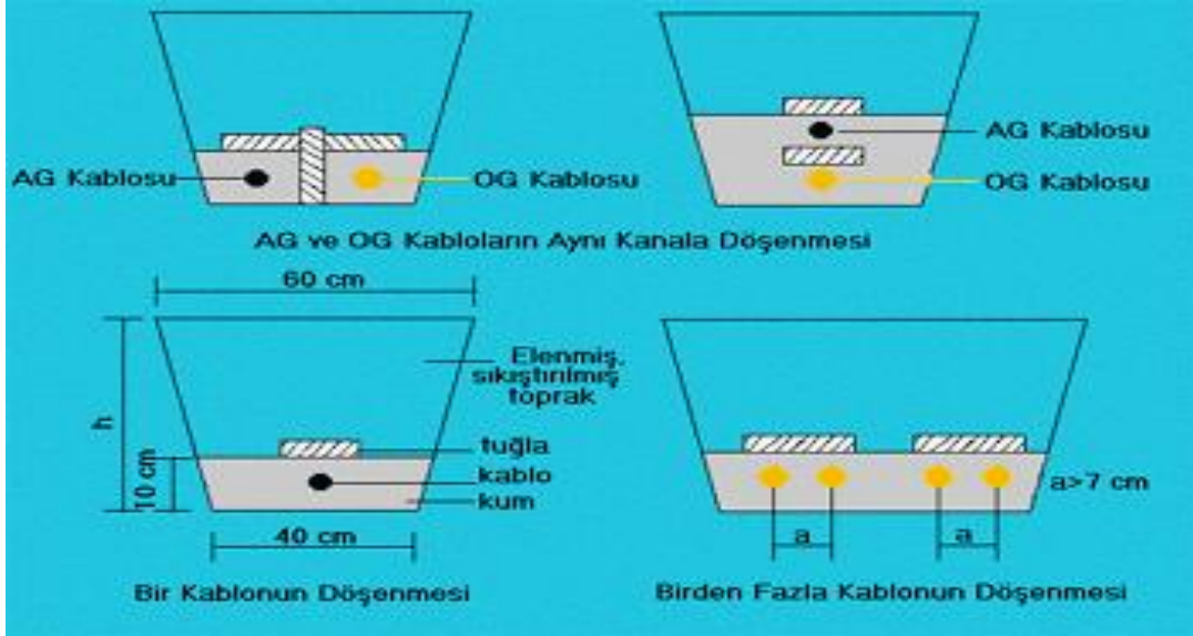
Şekil 2.12: Kablo kanalı özellikleri
