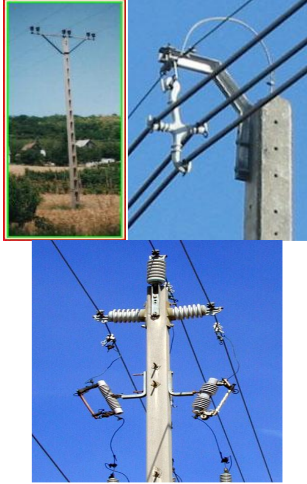
Resim 1.10: Vibre tip (VBA) beton direkler
