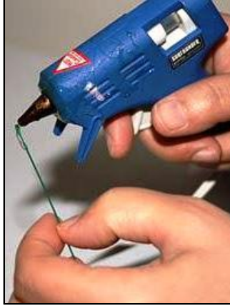
Resim 2.17: Yapıştırıcı tabancası kullanımı
