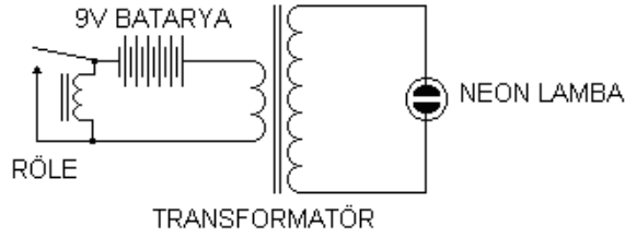
Şekil 4.1: Neon lamba bağlantı prensibi
