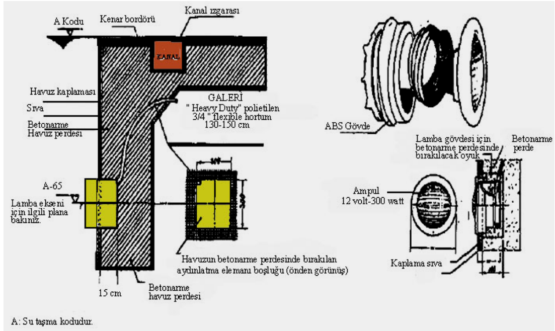
Şekil 5.1: Havuzun betonarme perdesindeki aydınlatma elemanı
