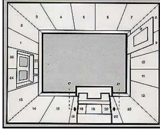
Resim 1.10: Kullanılacak duvar kâğıdı miktarının tespiti (oda üst görünüş)
