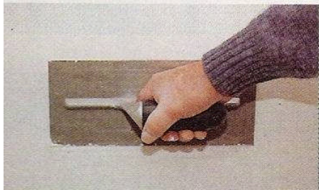
Resim 1.6: Yüzeye saten alçı perdah çekilmesi
