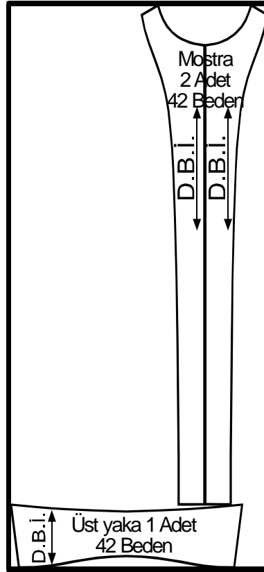
Şekil 2: Tela eni 90cm Tela kalıplarını açık enli olarak telaya yerleştirme
