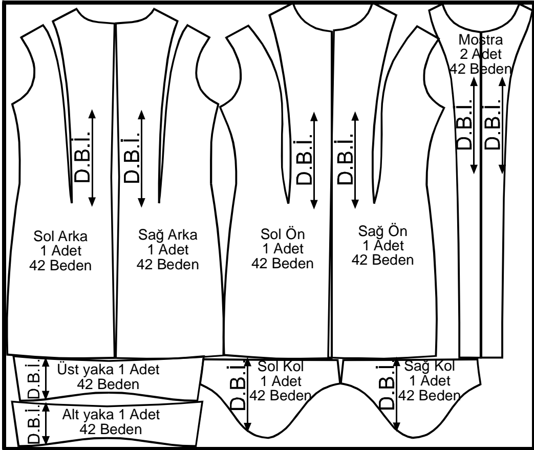
Kumaşın eni 150 cm Şekil. 1: Kalıpları açık enli olarak kumaşa yerleştirme
