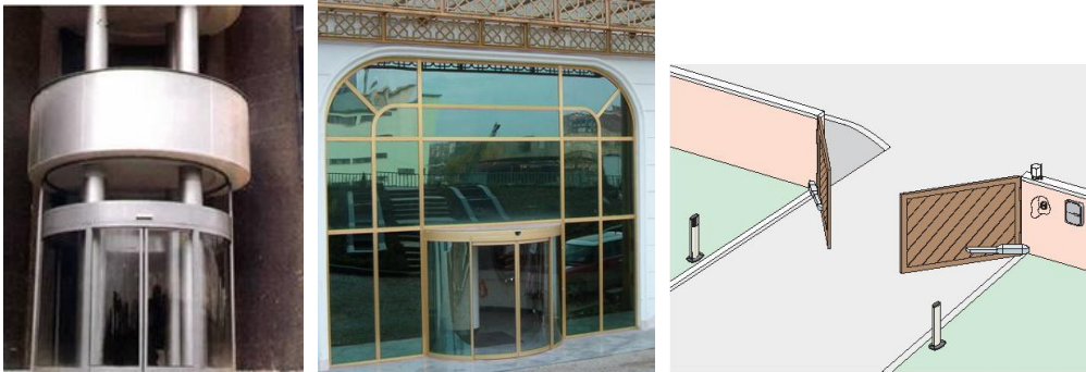
Şekil 3.2: Dairesel açılır kapılar
