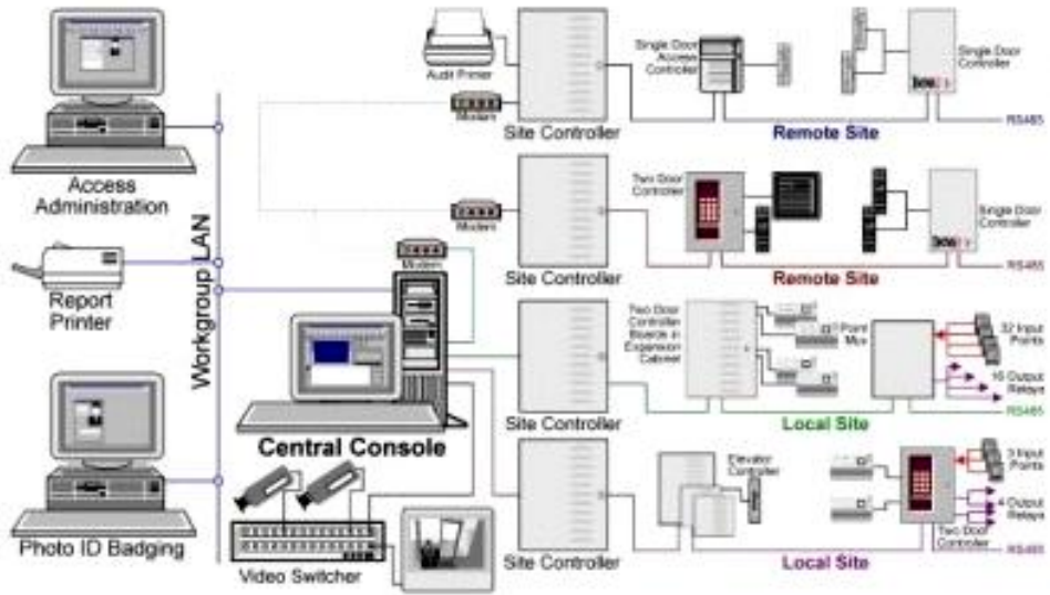
Şekil 3.17: PDKS blok şeması
