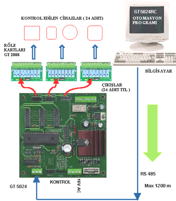
Şekil 2.4: Sistem bağlantıları
