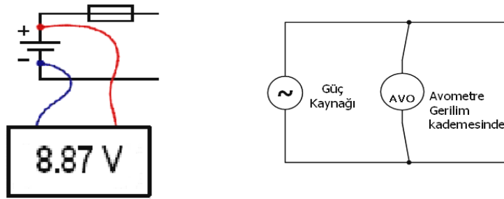
Şekil 1.4: Bir devrede gerilim ölçmek
