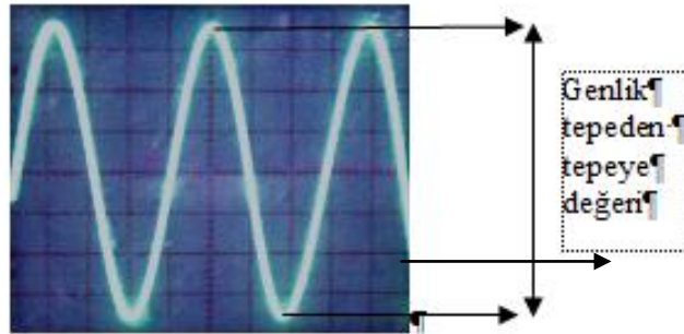
Şekil 1.10: Sinyalin genliği tepeden tepeye noktasıdır
