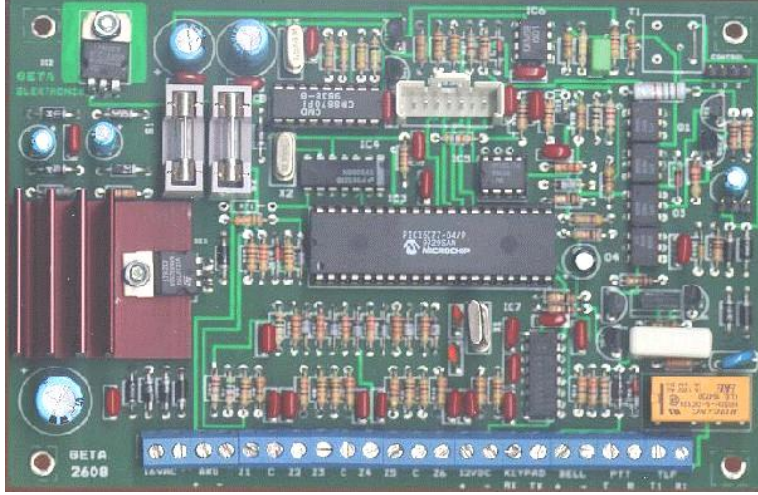
Şekil 1.2: Geçiş kontrol sistemini oluşturan kontrol kartlarından biri
