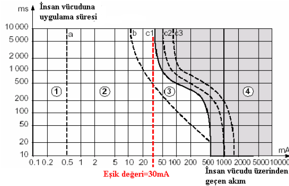
Şekil 1.11: IEC 60479-1'e göre AC akım etkileri
