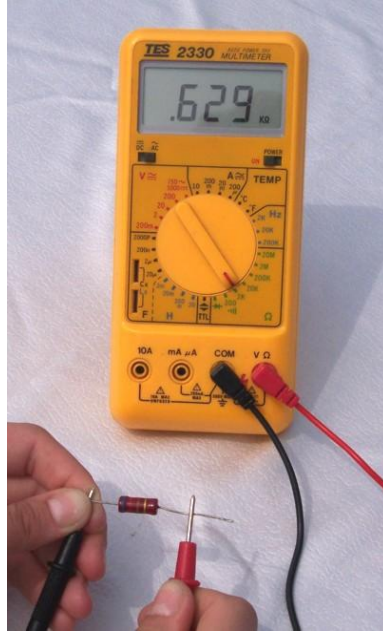
Şekil 1.5: Direnç ölçüm şekli
