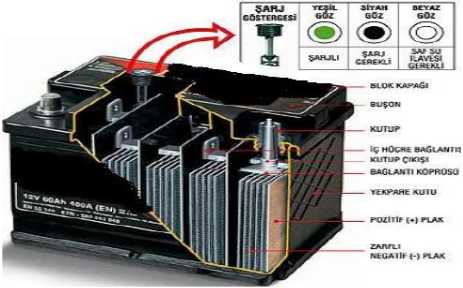
Şekil 3.1: Akümülatör yapısı
