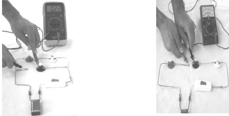
Şekil 1.3: Bağlantı yolları testi
