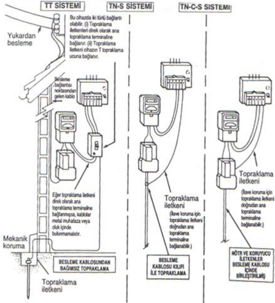
Şekil 1.14: Çeşitli topraklama sistemleri
