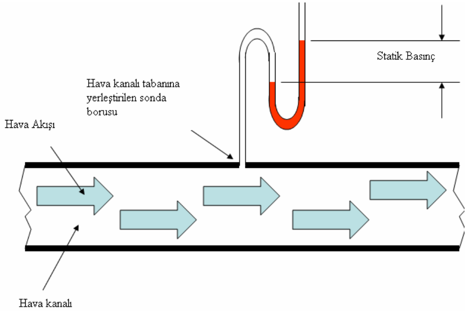
Şekil 3.4: Hava kanalı tabanına yerleştirilmiş boru
