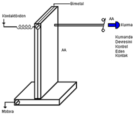
Şekil 1.4: Endirekt ısıtmalı termik
