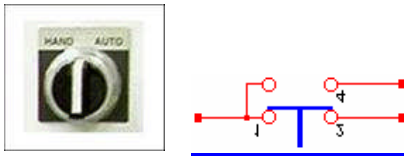
Resim 1.22: Çift yönlü buton
