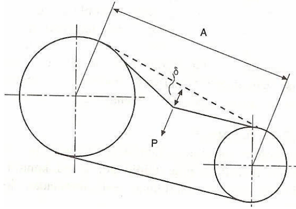
Şekil 2.10: Kayış gerginliği kontrolü
