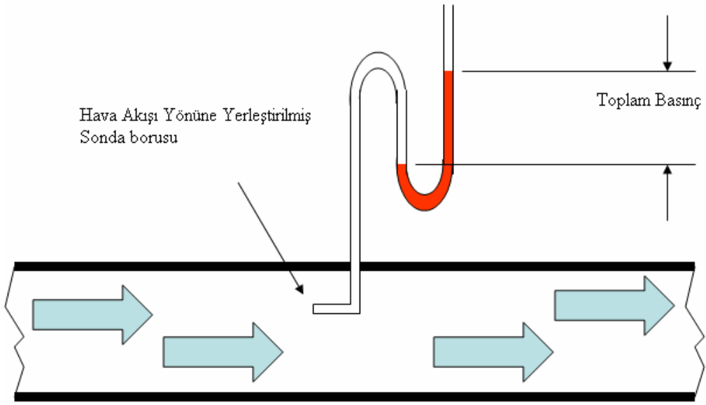
Şekil 3.3: Hava akış yönüne yerleştirilmiş boru
