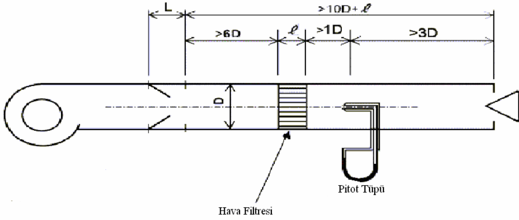
Şekil 3.7: Pitot tüpü ile hava kanallarında hız ölçümü
