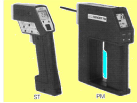
Resim 4.4: Işınım termometreleri
