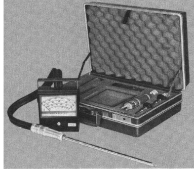
Resim 3.5: Velometre
