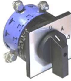
Resim 1.17: Yıldız üçgen pako şalteri
