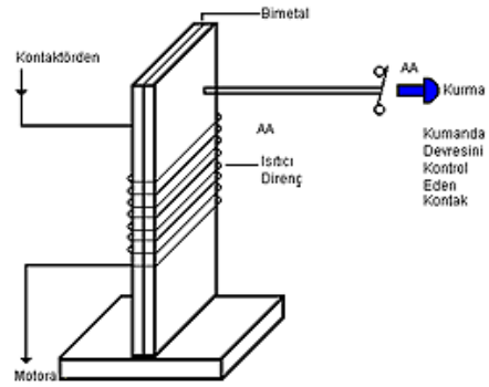
Şekil 1.5: Direkt ısıtmalı termik
