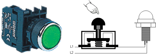
Resim 1.20: Kumanda butonu
