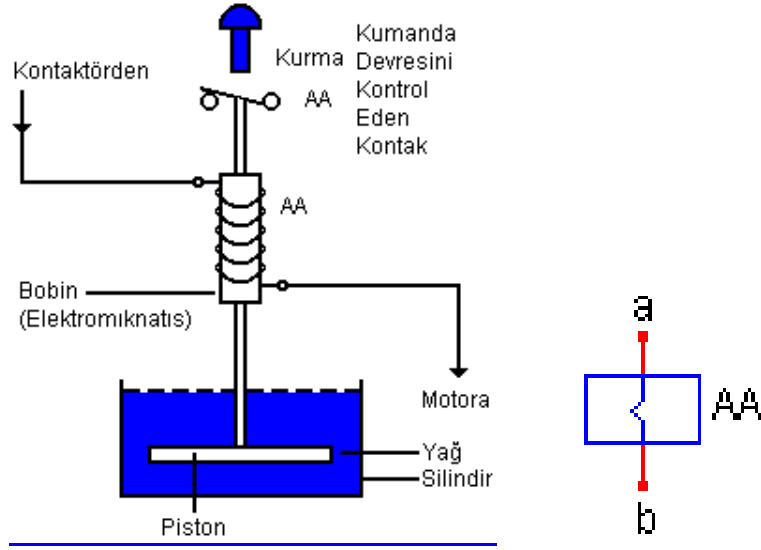
Şekil 1.3: Manyetik aşırı akım rölesinin iç yapısı ve sembolü
