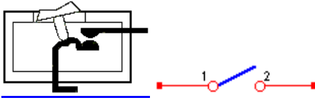
Şekil 1.2: Anahtarın iç yapısı ve sembolü
