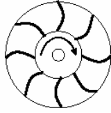
Şekil 2.6: Geriye eğimli kanat tip
