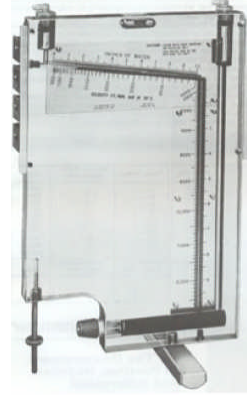
Resim 3.11: Eğimli ve dik manometre
