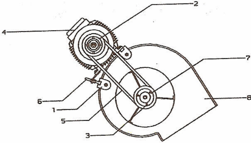
Şekil 2.9: Kayış-kasnak sistemi elemanları
