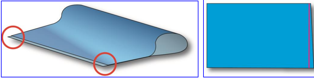
Şekil 1.20 : Kesim öncesi kontrol ve çarpıklığın düzeltilmesi için alınan tıraş
