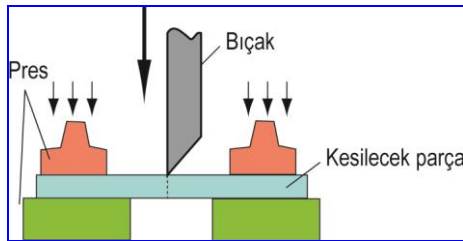
Şekil 1.8 : Patlatma kesim prensibi
