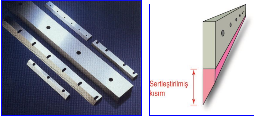
Şekil 3.12 : Bıçak
