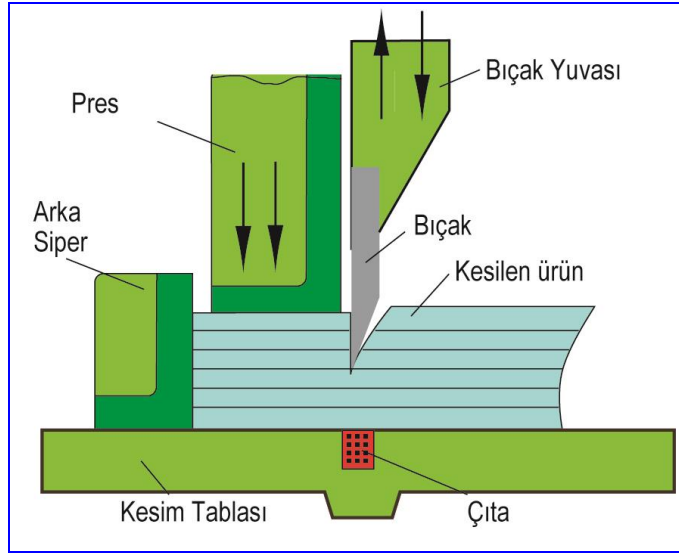
Şekil 3.13 : Giyotin kesim şeması
