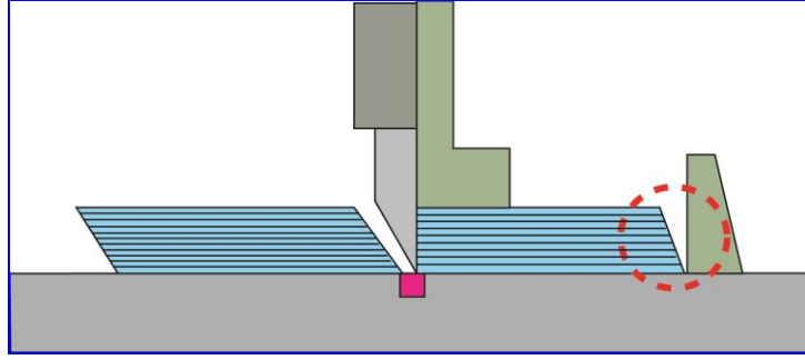
Şekil 3.23 : Bıçağın çekmesi
