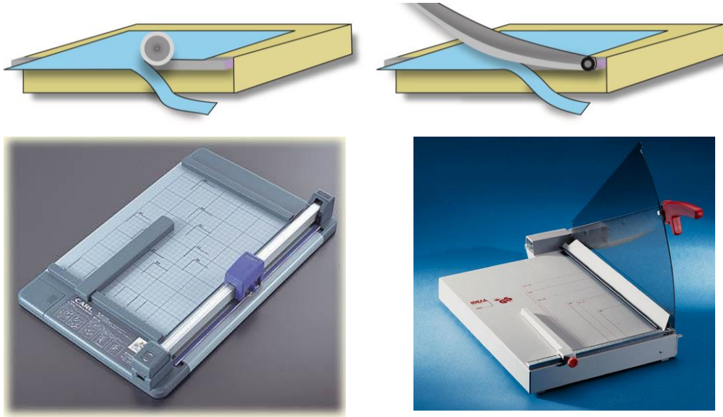
Şekil 2.3: Bıçaklarına göre kâğıt makası çeşitleri
