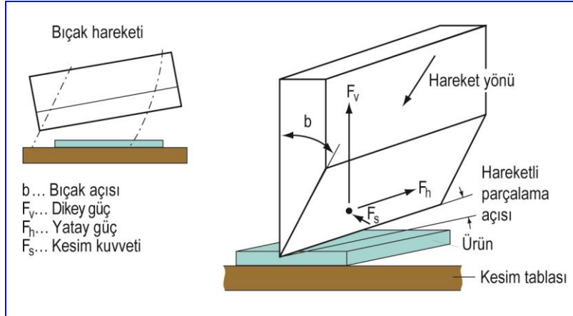
Şekil 3.14 : Giyotin kesim
