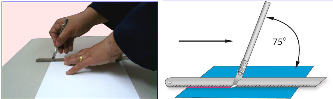
Şekil 1.14 : Tutuş şekli
