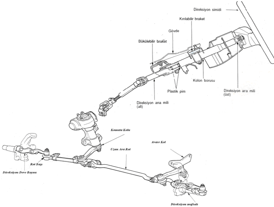
Şekil 3.10: Direksiyon sistemi
