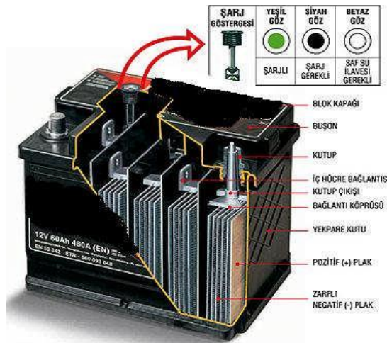
Şekil 4.1: Akü kesiti
