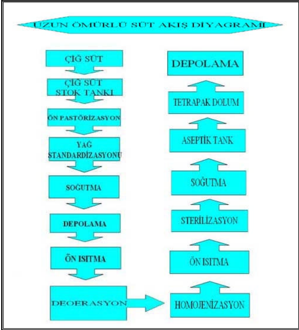
Resim 2.9: UHT süt akış diyagramı
