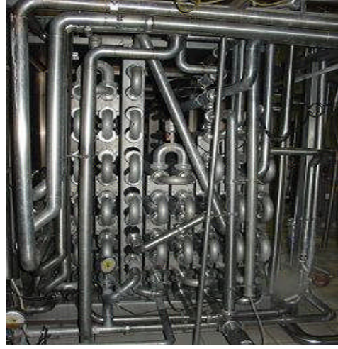
Şekil 1.6 ve Resim 1.2: Borulu ısı deđiřtiricinin genel görünümü
