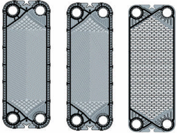
Şekil 1.4: HTST pastörizasyonunda kullanılan ısı değiştirici plaka modelleri
