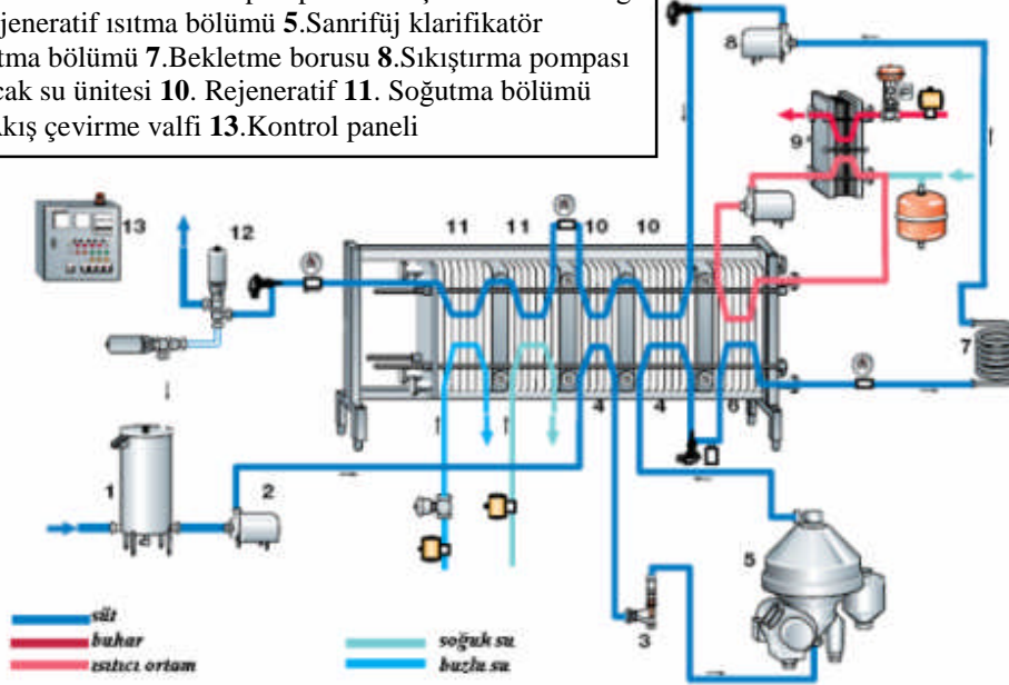
Şekil 1.5: Plakalı ısı deęiřtirici pastörizatörün kullanıldıęı bir süt iřletmesi
