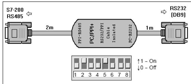
Şekil 1.1: PC/ PPI kablosu sviç konumları
