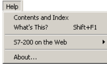
Şekil 2.35: Help menüsü
