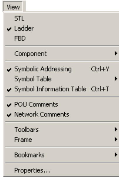
Şekil 2.24: View menüsü
