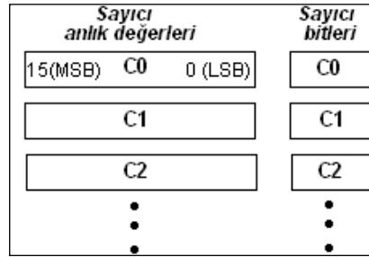
Şekil 2.58: Sayıcı adresleri
