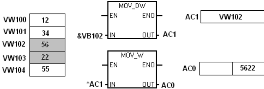
Şekil 2.59: Endirekt adresleme
