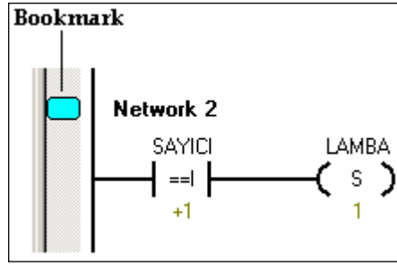
Şekil 2.29: Bookmark
