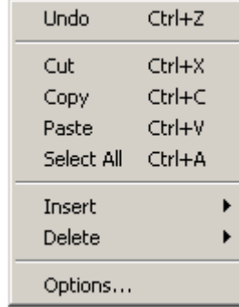
Şekil 2.36: PLC menüsü
