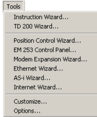
Şekil 2.33: Tools menüsü
