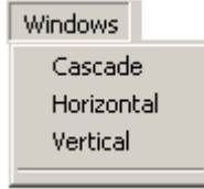
Şekil 2.34: Windows menüsü
