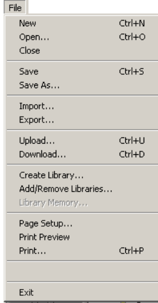
Şekil 2.21: File menüsü
