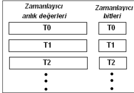
Şekil 2.57: Zamanlayıcı adresleri
