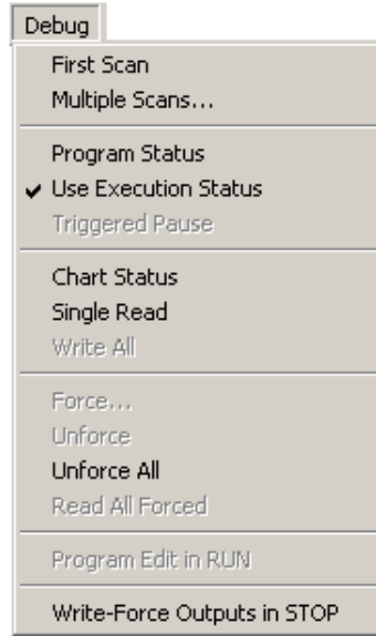
Şekil 2.32: Debug menüsü
