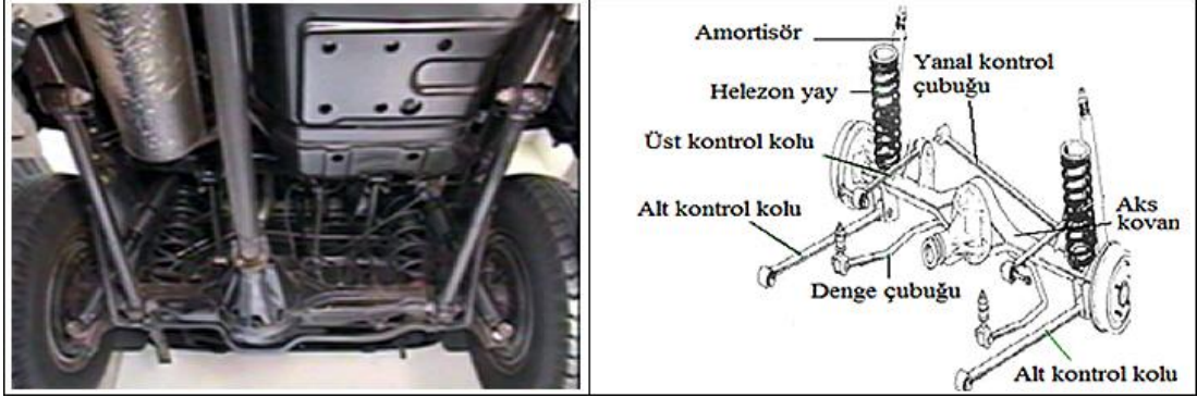
Resim 3.2: Dört bağlantılı sabit süspansiyon sistemi
