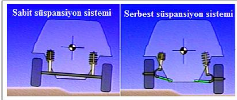
Şekil 3.1:Süspansiyon sistemi çeşitleri
