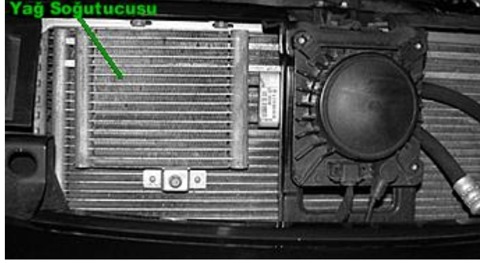
Resim 4.20: Yağ soğutucusu
