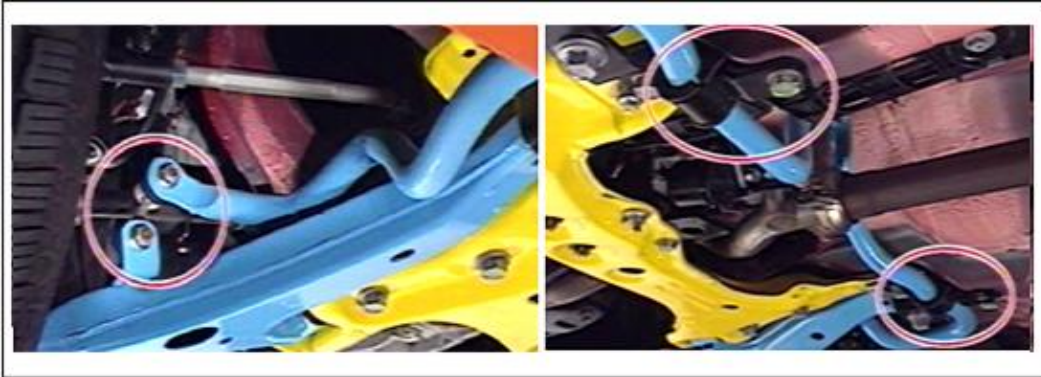
Resim 2.8: Denge çubuğunun bağlantıları
