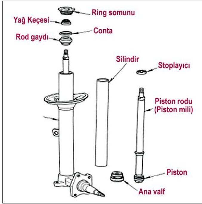
Şekil 1.15: Amortisörü oluşturan parçalar
