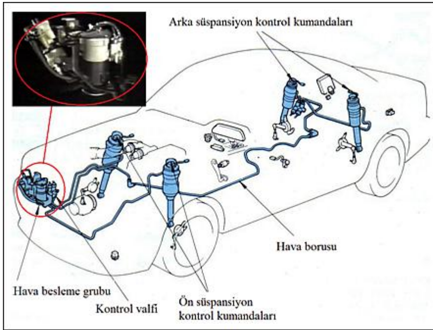
Şekil 4.6: Aktif kontrollü havalı süspansiyon sistemi ve hava besleme bölümü
