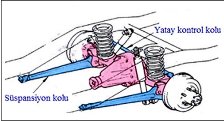
Şekil 3.5: Yatay kontrol kollu helezon yaylı sabit arka süspansiyon sistemi
