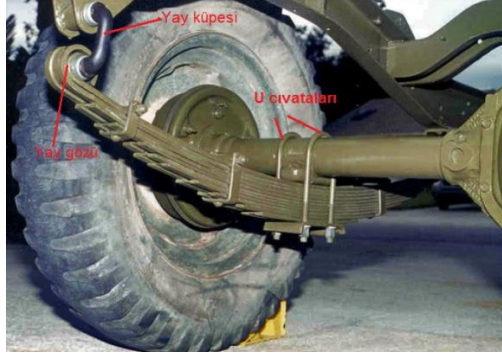
Resim 2.2: Yaprak yaylı süspansiyon sistemi
