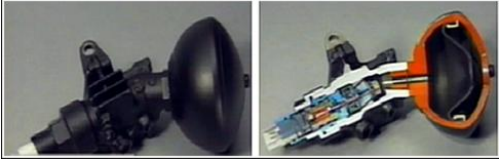
Resim 4.27: Gaz odası ve sönümlenme kuvveti kontrol kumandası
