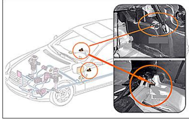
Resim 4. 11: Enlemesine ve boylamasına hızlanma sensörleri
