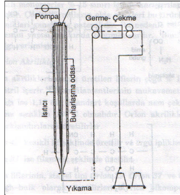
Şekil 2.1. Kimyasal Lif Eğirme
